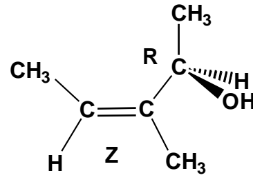
(2R,Z)-3-méthylpent-3-én-2-ol
