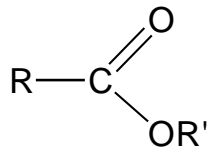
Ester
