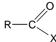
Halogénure d'acide
