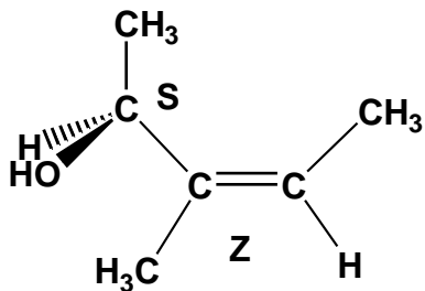
(2S,Z)-3-méthylpent-3-én-2-ol
