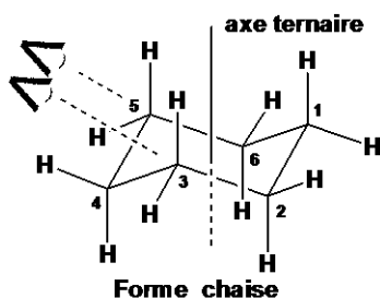
Forme chaise
